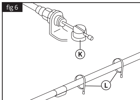
K. Recessed hole / Εγκοπή L. Bands / Κλιπς
