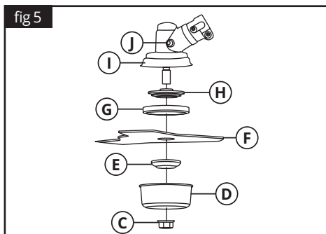
C. Nut / Βίδα D. Plate housing / Περιβλήμα πλάκας E. Low plate / Κάτω πλάκα F. 3T Blade / Λεπίδα 3T G. Adapter housing / Περιβλήμα προσαρμογέα H. Upper plate / Επάνω πλάκα I. Gear housing / Κέλυφος γραναζιών μετάδοση J. Hole / Οπή
