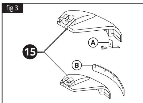
A. Cord cutter / Κόφτης μισινέζας B. Guard extension / Επέκταση προφυλακτήρα
