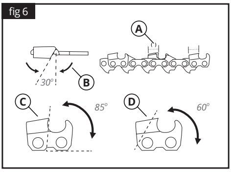
A. Cutter length / Μήκος λεπίδας B. Filing angle / Γωνία λείανσης C. Side plate angle / Γωνία πλευρικής πλάκας D. Top plate cutting angle / Γωνία πάνω πλάκας
